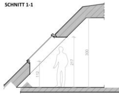
SCHNITT 1-1
