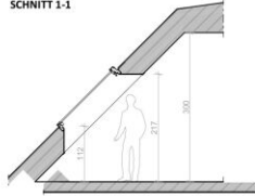
SCHNITT 1-1
